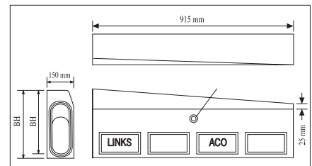
Lejtő elem
